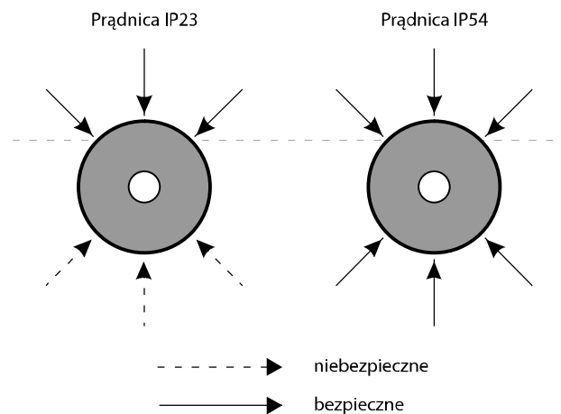
Rys.1 Opis oznaczeń stopnia ochrony IP
